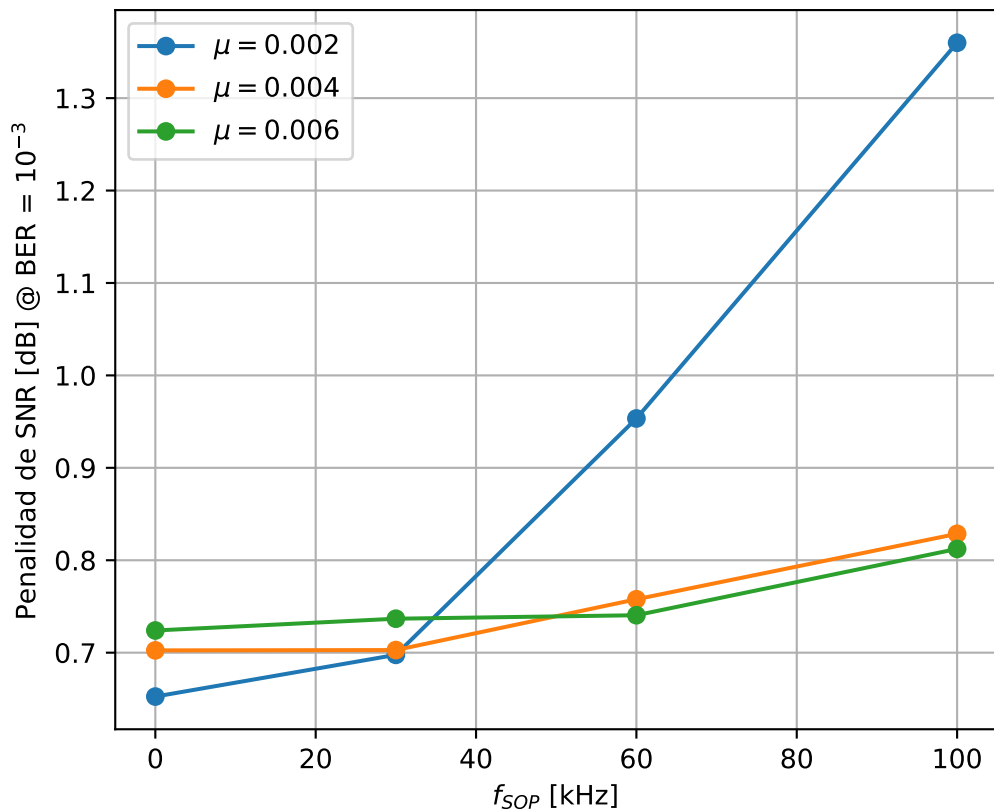
Penalidad de SNR debido a la rotación del SOP
